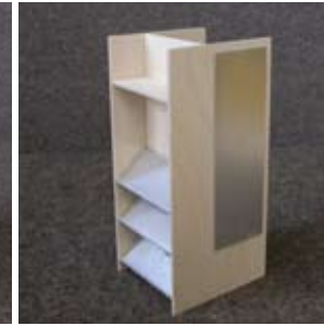
Rückseite von E/GA//QD mit Tablar und drei Schrägtab- laren
