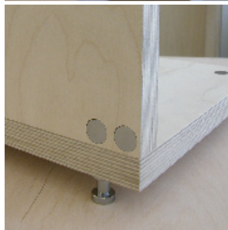
Beschlag als regulierbarer Stellfuss
