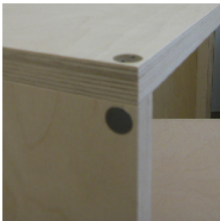
Verbindung einer liegenden und einer stehenden Platte
