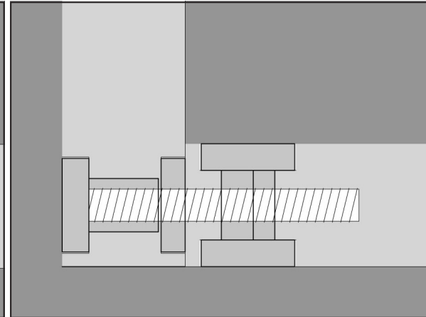
3. der Gewindestift ZH/GS
