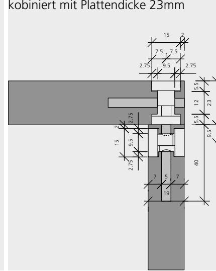
Bohrungen bei von Plattendicken 19mm kobiniert mit Plattendicke 23mm
