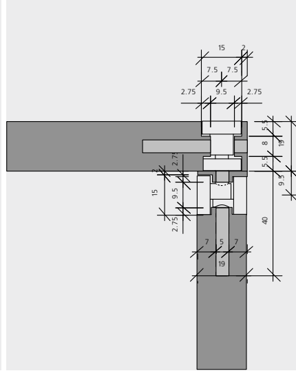
Bohrungen bei Plattendicke 19mm
