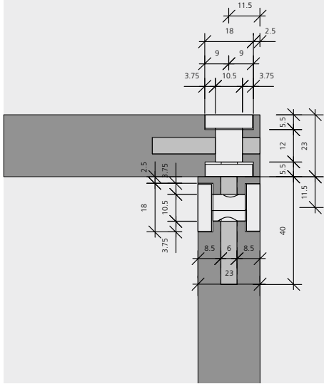
Bohrungen bei Plattendicke 23mm
